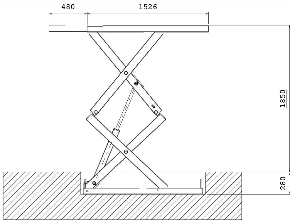
Sez. E-E
