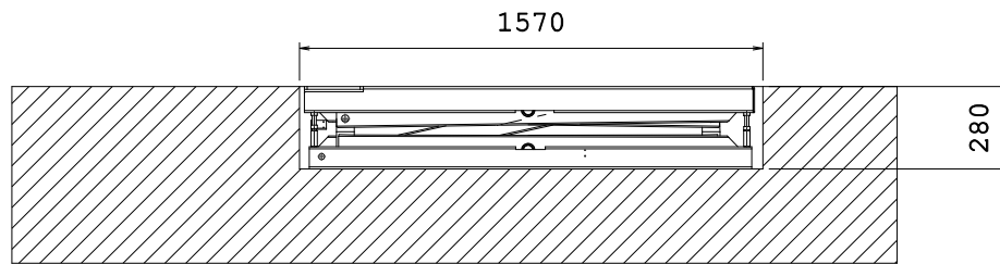
Sez. D-D
